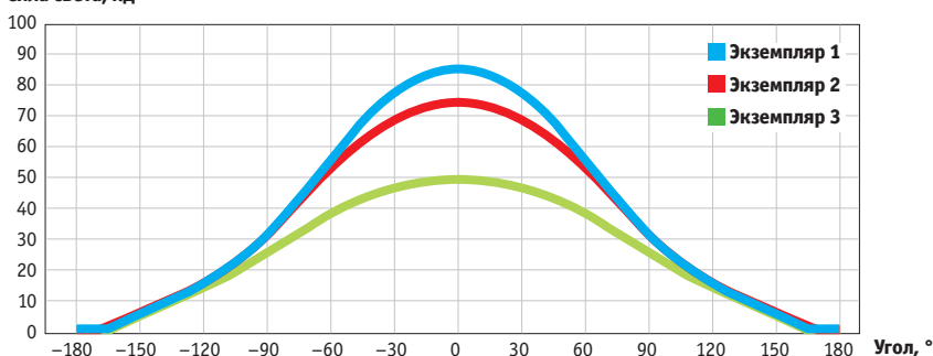
Сила света, кд
