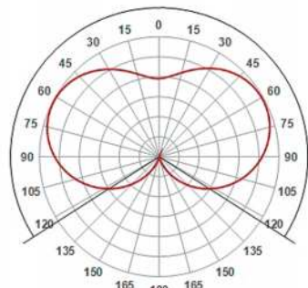
Яркость в зависимости от угла излучения
