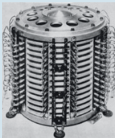
Drum Memory — «дедушка» жесткого диска
